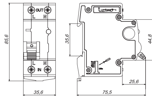
Рис. 3. Размеры УЗДП
