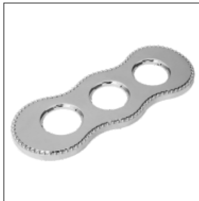
Рамка трехместная восьмерка Материал: металл Размер: 264x98x11 мм Цвет: хром BF8-630-30
